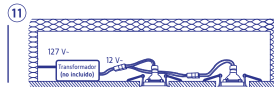
Diagrama para instalar una lámpara a 12 V-
