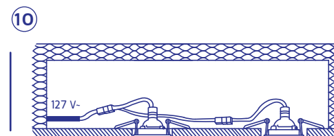
Diagrama para instalar una lámpara a 127 V-
