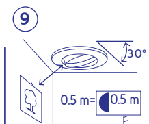
Distancia mínima de montaje
